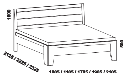
1005 / 1105 / 1705 / 1905 / 2105 postel SAGITA - šikmé nohy 90, 100, 160, 180, 200 x 200, 210, 220
