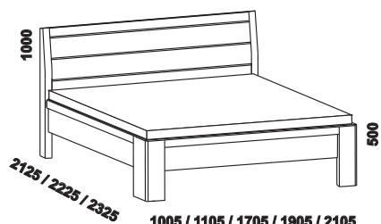
1005 / 1105 / 1705 / 1905 / 2105 postel SAGITA - rovné nohy 90, 100, 160, 180, 200 x 200, 210, 220
