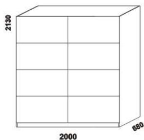
2130 2000 680 skříň š. 200 s posuvnými dveřmi – dělené dveře plné
