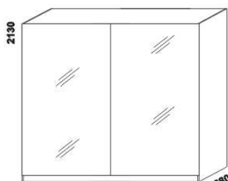
2130 2519 680 skříň š. 250 s posuvnými dveřmi – zrcadlové dveře
