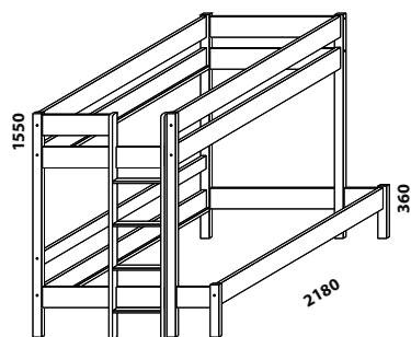
1290 EVISA etážová postel 90/120 × 200
