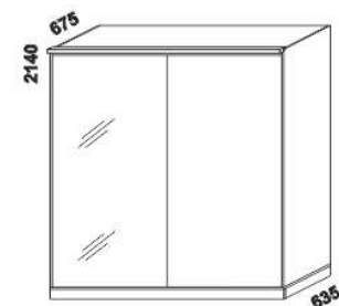
1524 / 2000 / 2516 skříň š. 150, 200, 250 s posuvnými dveřmi – dveře kombi plné / zrcadlové
