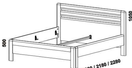
postel ENYA, čelo 2 – s příčkou 90, 120 x 200, 210, 220 140, 160, 180, 200 x 200, 210, 220
