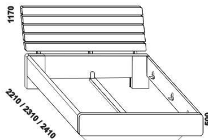
980 / 1080 / 1280 / 1480 / 1680 / 1880 postel LOREN, podnoží - sokl 90, 100, 120 x 200, 210, 220 140, 160, 180 x 200, 210, 220
