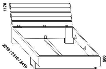
980 / 1080 / 1280 / 1480 / 1680 / 1880 postel LOREN, podnoží - ližina 90, 100, 120 x 200, 210, 220 140, 160, 180 x 200, 210, 220
