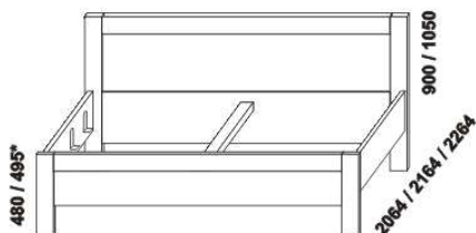
990 / 1284 / 1484 / 1684 / 1884 postel LINE, čelo 1 - plné 90, 120, 140, 160, 180 x 200, 210, 220
