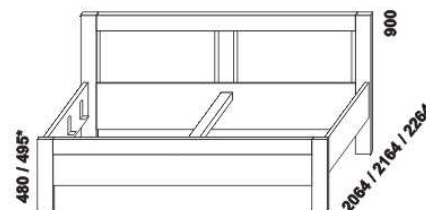
990 / 1284 / 1484 / 1684 / 1884 postel LINE, čelo 3 - dělené 90, 120, 140, 160, 180 x 200, 210, 220
