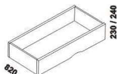
1600 / 1960 zásuvka boční 3/4 nebo celá
