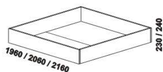
1600 / 1800 / 2000 úložný prostor Max 160, 180, 200 x 200, 210, 220
