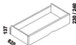
1600 / 1960 zásuvka boční pro motorové polohování 3/4 nebo celá
