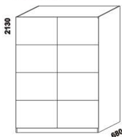
2130 / 1528 / 680 skříň š. 150 s posuvnými dveřmi - dělené dveře plné
