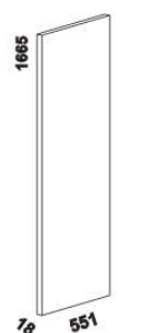
dělící příčka svislá
