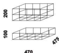
drátěný koš v. 20 nebo 10
