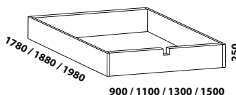
900 / 1100 / 1300 / 1500
