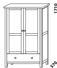
900 šatní skříň
