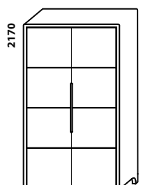
1200 skříně 2dveřová
