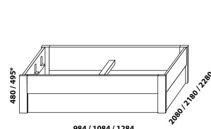
984 / 1084 / 1284 1484 / 1684 / 1884 / 2084
