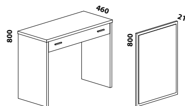
1050 toaletní stolek
