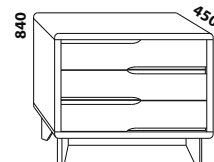
1000 komoda 3zásuvková
